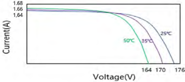
COM-Z3-T30不同温度下的IV曲线
