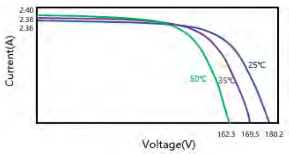
COM-M2-280W不同温度下的IV曲线
