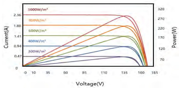
COM-M2-280W不同光强下的IV曲线
