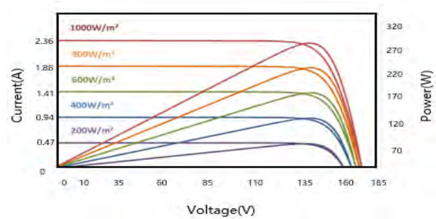
COM-M1-280W不同光强下的IV曲线
