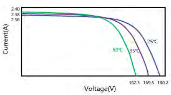
COM-M1-280W不同温度下的IV曲线
